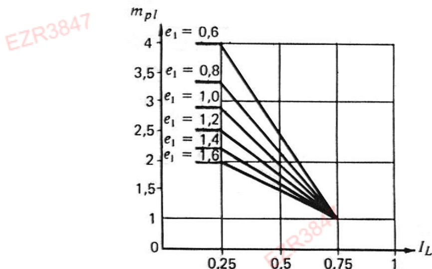
Рисунок В.1 – График для определения коэффициента m_{pl}
