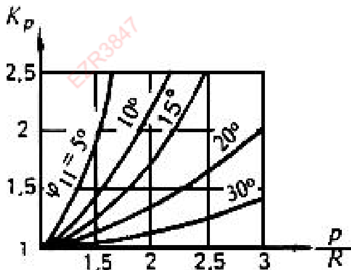
Рисунок Л.1 – График для определения коэффициента K_p
