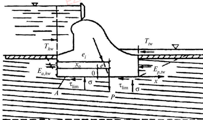
Рисунок Г.2 – Схема к расчету устойчивости сооружения на сдвиг по плоской поверхности основания с неоднородной поперечной слоистостью грунтов при малом угле падения слоев
